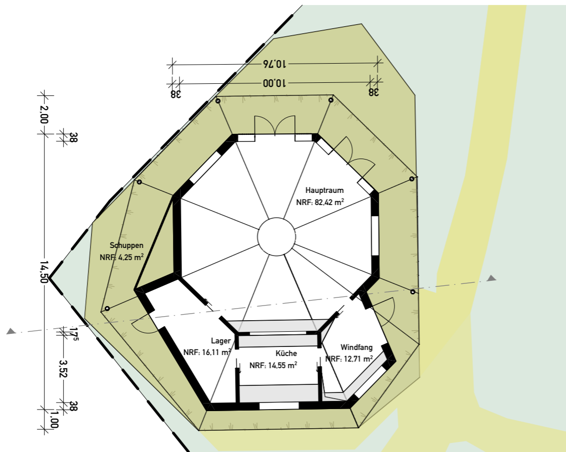
Grundriss 1:200
