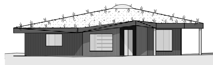
A-01 Ansicht Nord 1:200
