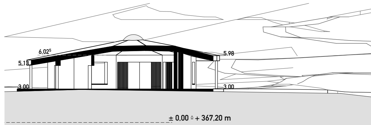
Schnitt 1:200
