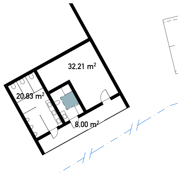
UG-Grundriss
