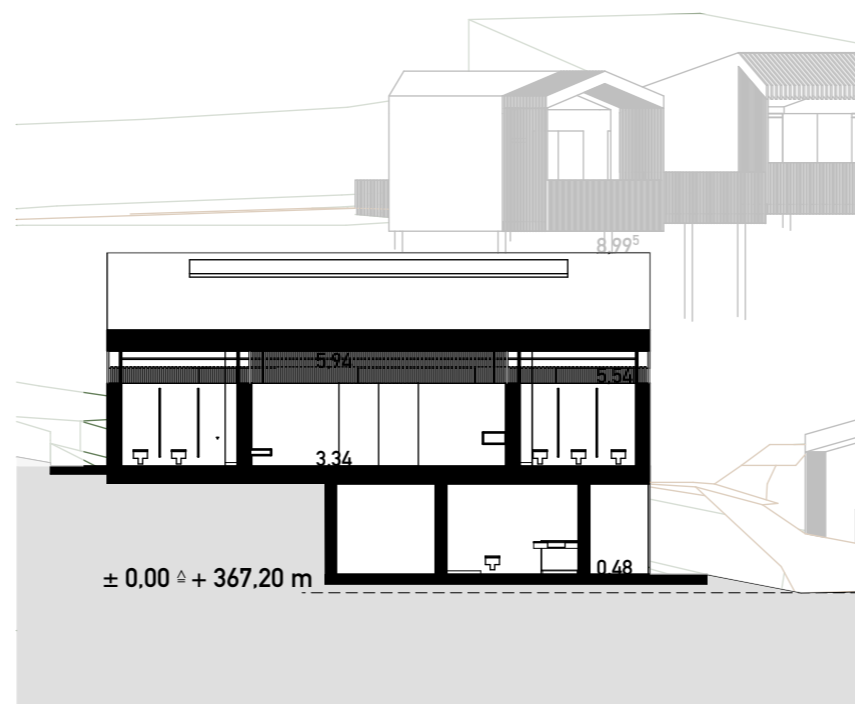
Längs-Schnitt
